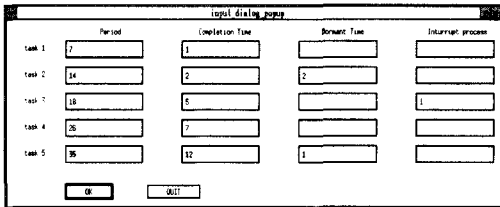
(그림 15) 태스크 집합의 입력 데이터 (II)
