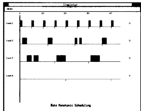
(그림 13) 비율 단조 스케줄링 시뮬레이션 결과 (1)
