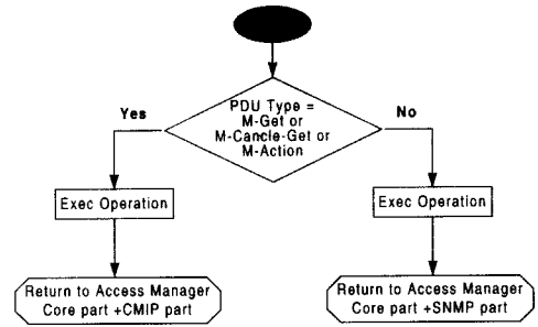
(그림 12) GP(General Procedure)의 처리 알고리즘
