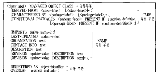
(그림 2) 확장된 Managed Object Class 템플릿
