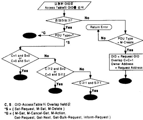
(그림 11) Access Manager의 처리 알고리즘
