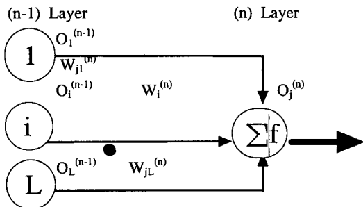
그림 3.1 (n) th Layer의 Neuron Model
