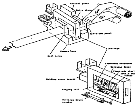
그림 4.1 MESH SEAM WELDER의 구조
