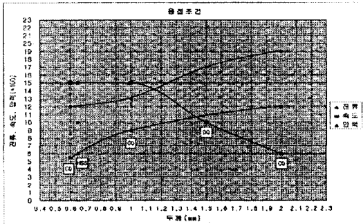
그림 4.3 정상 조업시 얻어진 용접조건
