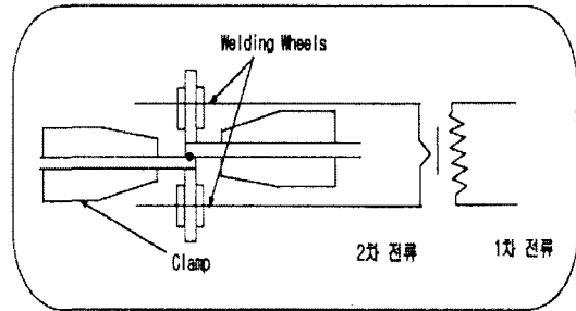
그림 4.2 Welder의 동작원리
