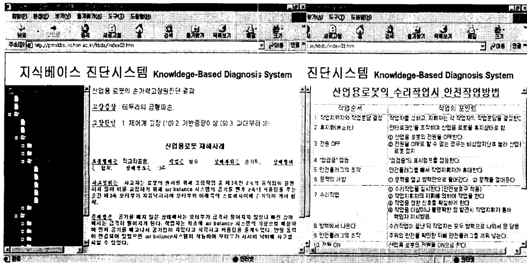
<그림 12> 산업용 로봇 핸드부분 고장원진단 결과화면
