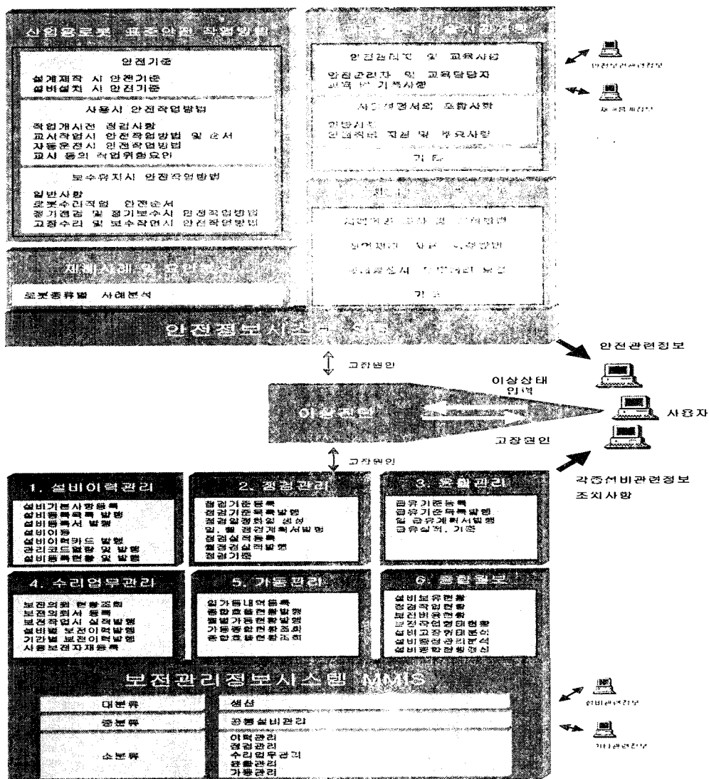
<그림 4> SIS와 MMIS 및 지식베이스 진단시스템의 정보흐름도
