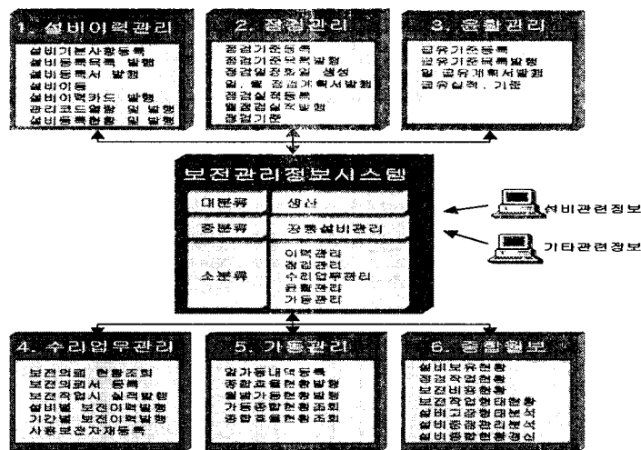
<그림 8> 보전정보시스템의 구성도
