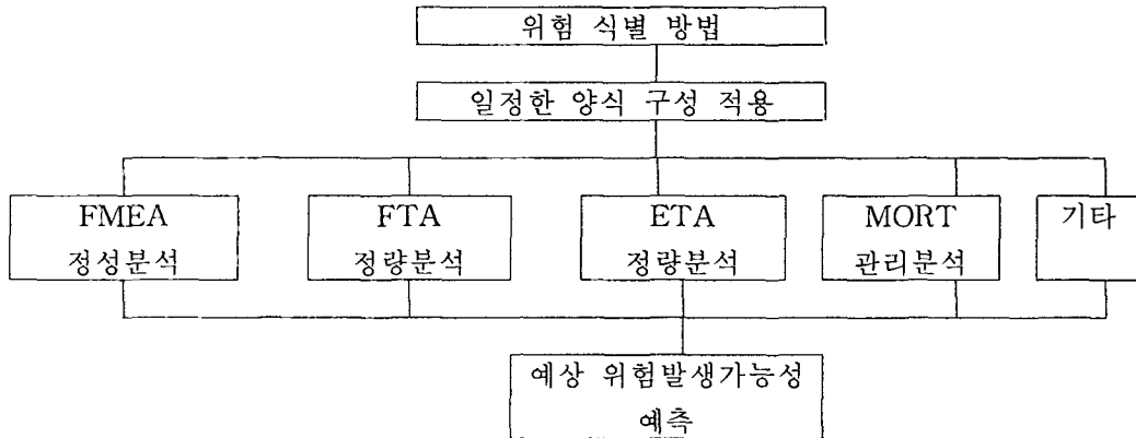
<그림 4> 위험식별 확인방법
