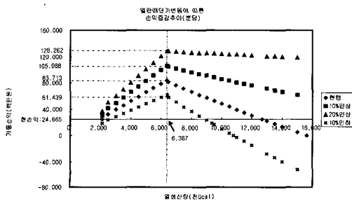
<그림 8> 열판매단가변동에 따른 손익증감추이
