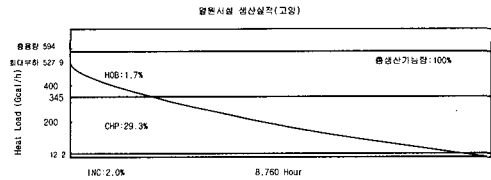
〈그림 7〉 열원시설 생산실적
