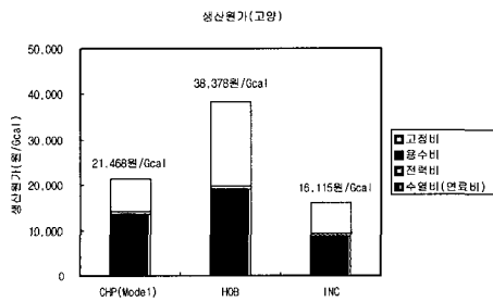
〈그림 6〉 열원별 생산원가
