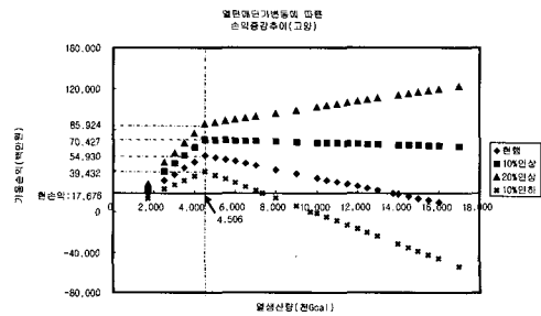
<그림 8> 열판매단가변동에 따른 손익증감추이
