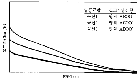
〈그림 5〉 열공급량 증가에 따른 CHP생산량 변동
