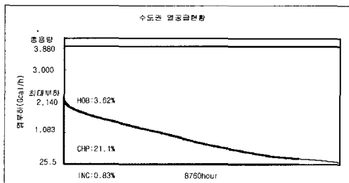
〈그림 2〉 수도권 열공급 현황
