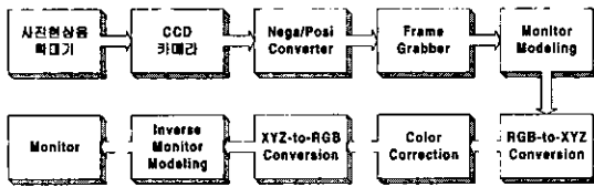
그림 3. 시스템 구성도
