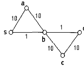
그림 3. 망 토폴로지
