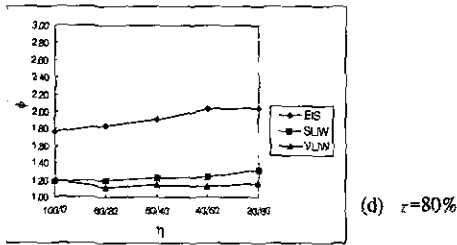
그림 9. 자료중속성 비율의 변화에 따른 성능 비교
