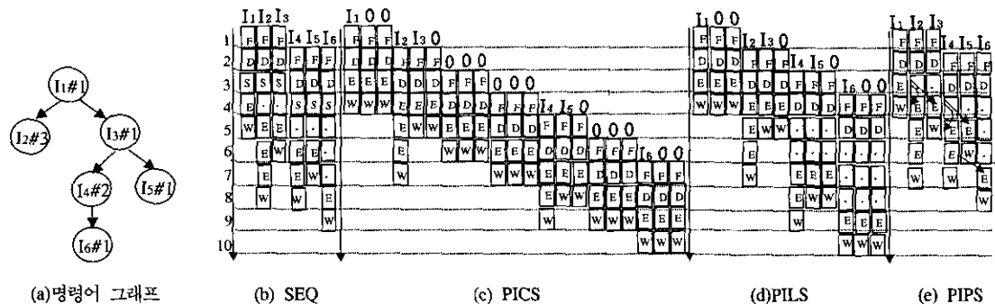
그림 2. 프로세서 구조별 명령어실행 흐름
