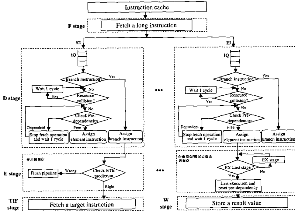
그림 6. 명령어 파이프라인 과정
