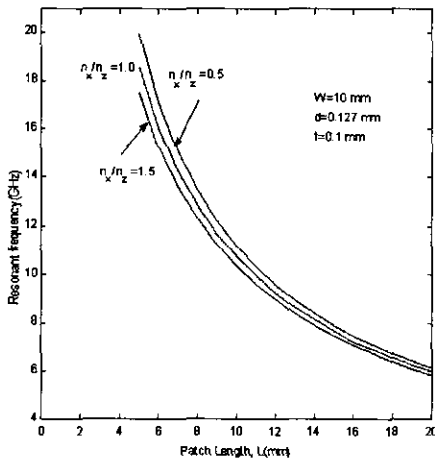
그림 4. W=10\text{mm} 일때의 이방성 비( \epsilon_z = 2.35 )에 대해 L 의 길이의 변화에 따른 공진주파수
