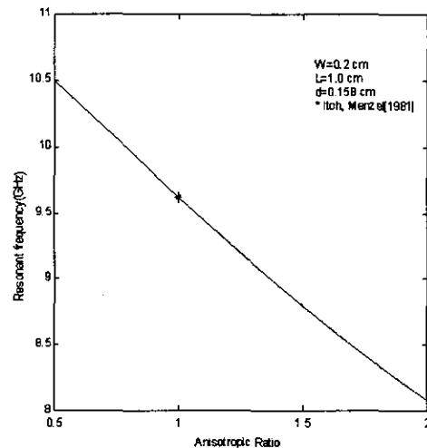
그림 2. 공기 갭의 두께가 0 일 경우 본 논문의 결과와 [1]의 논문에서의 결과 비교
