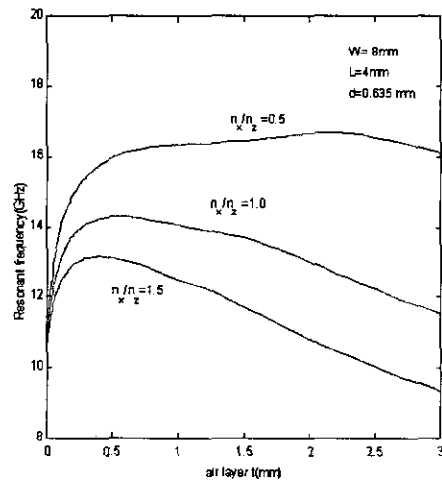
그림 5. W=8\text{mm} L=4\text{mm} 일때의 이방성 비( \epsilon_z = 9.6 )에 대해 공기 갭의 변화에 따른 공진주파수
