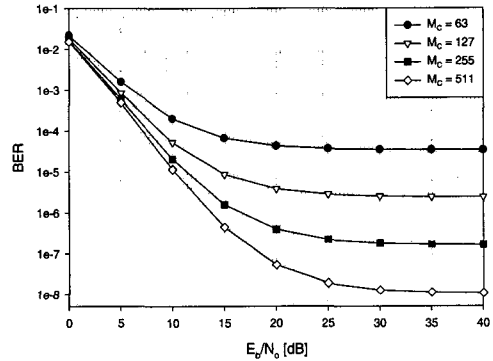
그림 6. 주파수 선택성 다중경로 페이딩 채널에서 Multi-Carrier의 수에 따른 Multi-Carrier CDMA 시스템의 오율 성능 ( \beta = 0.1 , 다중접속 사용자수=26, 다중사용자 간섭분포 : Case I, RAKE 수신기의 가지수=4 )
