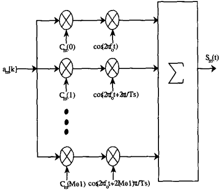
그림 3. Multi-Carrier CDMA 시스템의 송신기 구조
