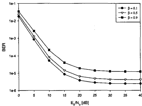
그림 5. 주파수 선택성 다중경로 페이딩 채널 특성( \beta )에 따른 Multi-Carrier CDMA 시스템의 오율 성능 (다중사용자 수=26, Multi-Carrier의 수=127, 다중사용자 간섭분포 : Case I, RAKE 수신기의 가지수=4 )
