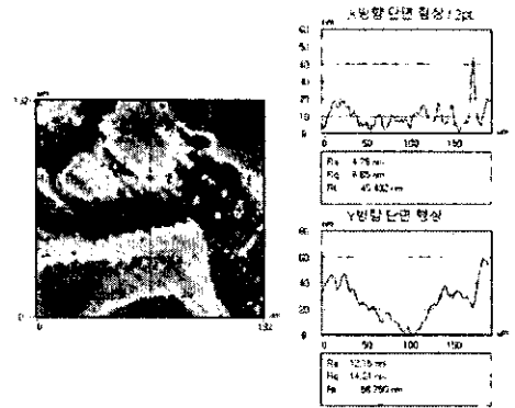
(d) TMAH 20 wt.%.
