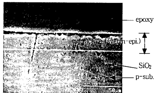
그림 4. 전기화학적 식각정지에 의해 제작된 SDB SOI기판의 단면 SEM사진.
