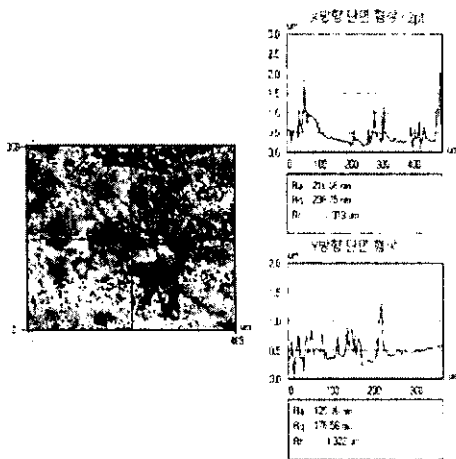
(b) TMAH 10 wt.%.
