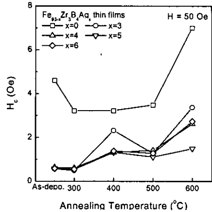
그림 5 열처리 온도에 따른 Fe_{93-x}Zr_3B_4Ag_x ( x=0, 3, 4, 5, 6 at.%) 박막의 보자력( H_c ) 변화.
