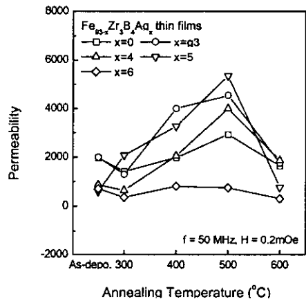
그림 6 열처리 온도에 따른 Fe_{93-x}Zr_3B_4Ag_x ( x=0, 3, 4, 5, 6 at.%) 박막의 투자율( \mu ) 변화.
