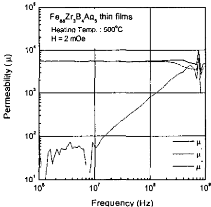
그림 7 500°C 열처리한 Fe_{88}Zr_3B_4Ag_5 박막의 투자율-주파수 의존성.
