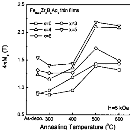
그림 4 열처리 온도에 따른 Fe_{93-x}Zr_3B_4Ag_x ( x=0, 3, 4, 5, 6 at.%) 박막의 포화자화( 4\pi M_s ) 변화.
