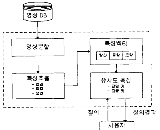
그림 6. 특징벡터 구성과 질의 수행 과정
