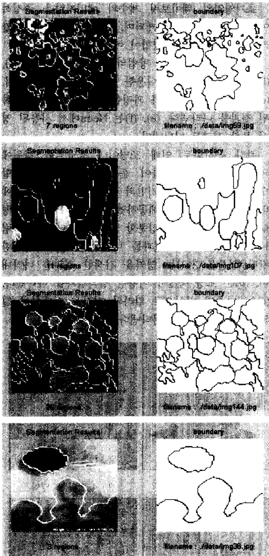
그림 11. 영상 분할결과
