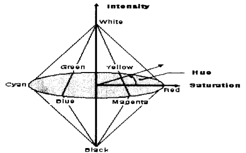
그림 2. HSI 좌표계
