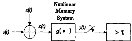
그림 1. 단순 등가 기저대역 통신시스템 구성도
