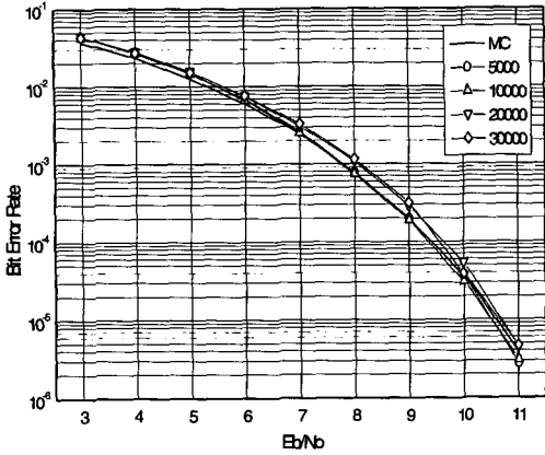
(b) TWTA의 input back-off가 -1dB일 때
