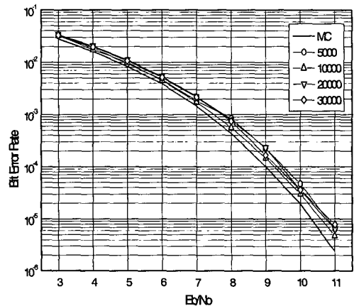
(a) TWTA의 input back-off가 -14dB일 때
