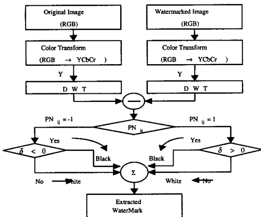
그림 3. 워터마크 검출 알고리즘
