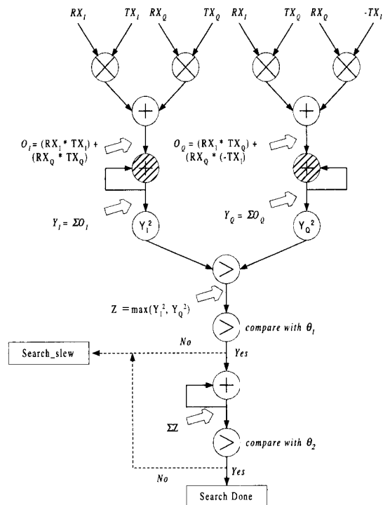
그림 5. 분할된 탐색자의 data flow graph
