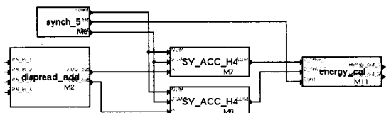
그림 14. 에너지 계산 블록
