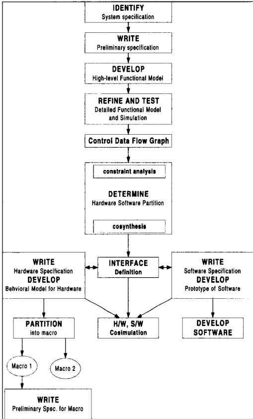
그림 1. 하드웨어-소프트웨어 통합설계의 전체 흐름도
