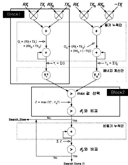
그림 3. 탐색자의 data flow graph
