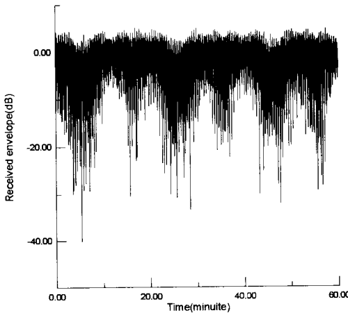
그림 6. 전원지역에서 양각의 변화에 대한 페이딩 크기.
