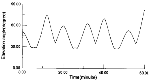
그림 4. Globalstar의 양각의 변화.
