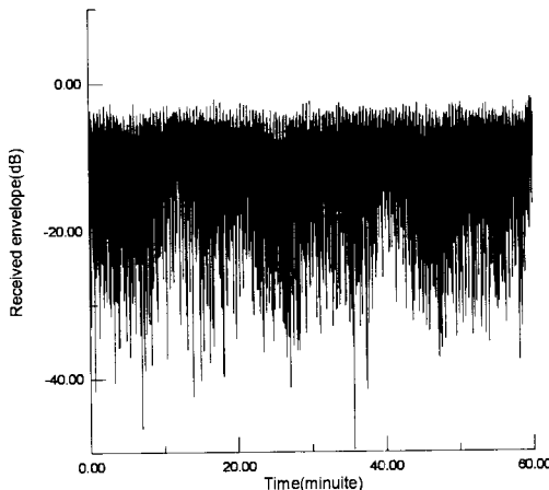
그림 7. 도심지역에서 양각의 변화에 대한 페이딩 크기.
