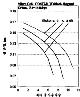
그림 14. 사용자 수에 따른 셀 반경 곡선 ( P_{rel}=0.8 )
