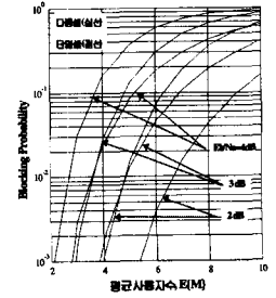
그림 12. Blocking 확률 곡선 (마이크로셀, X_0=0.9 )
