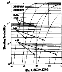
그림 11. Blocking 확률 곡선 (매크로셀, X_0=0.9 )
