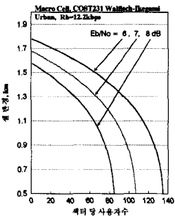
그림 13. 사용자 수에 따른 셀 반경 곡선 ( P_{rel}=0.8 )
