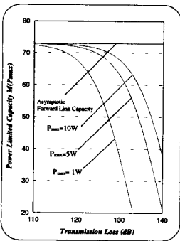
그림 2. 전송손실과 전송전력에 따른 시스템 용량
