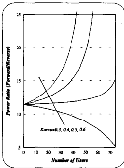
그림 5. 순방향-역방향의 전력비(음성)
