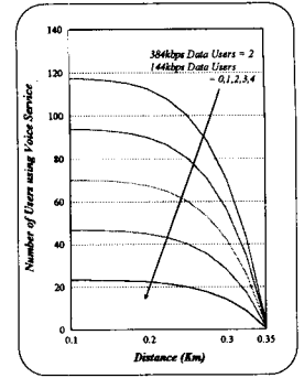
그림 18. 다양한 서비스에 대한 마이크로 셀에서의 용량
