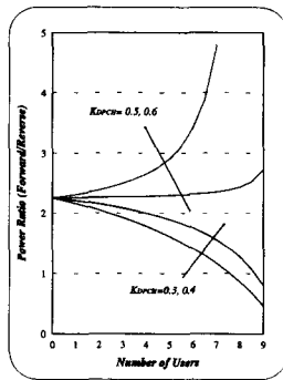
그림 6. 순방향-역방향의 전력비(데이터)
