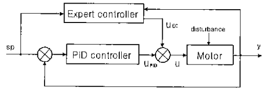
그림 1. PID-전문가 복합형 제어기를 갖는 시스템 구성도
