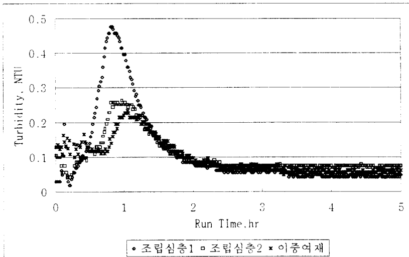
그림 2. 여층구성별 초기탁질 누출특성 비교
