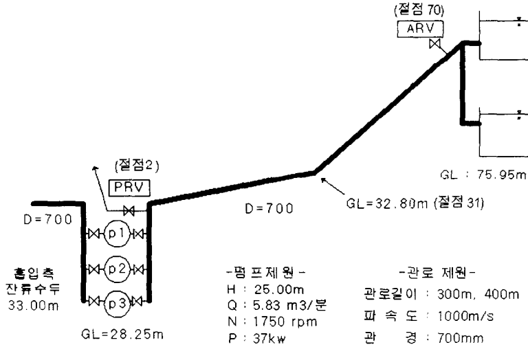
그림 3. 서변 펌프가압장
