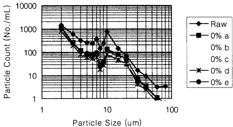
그림 3 트라프 폐쇄전 처리수 입도분포
