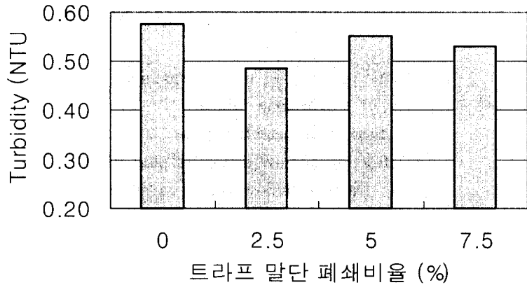
그림 2 트라프 폐쇄 후의 처리수 탁도
