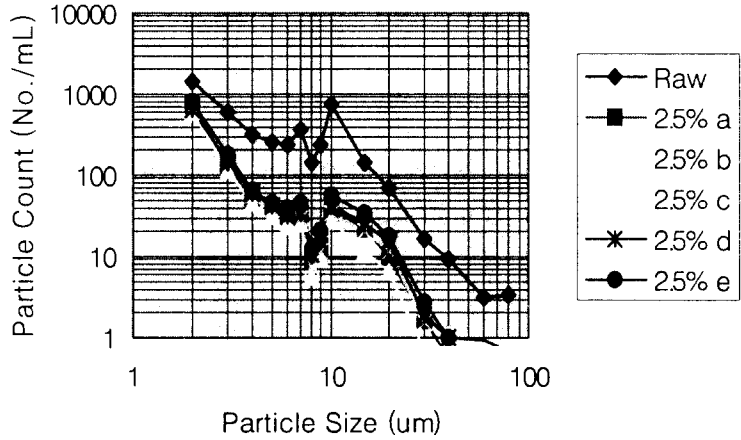
그림 4 트라프 2.5% 폐쇄시 침전지처리수 입도분포
