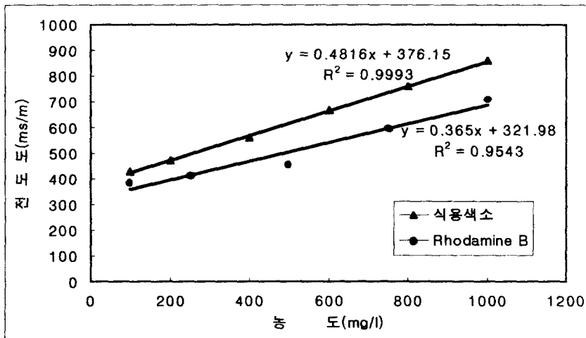
그림 3. 전도도-농도 곡선
