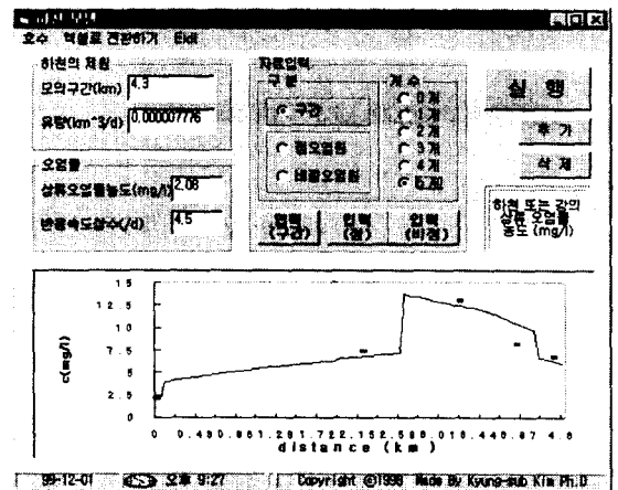
그림 2.2.3 하천모델
