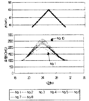
그림 7 수로내 각 단면의 유량변화
