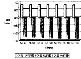
그림 19 합류점 이후에서의 유속비교(최소값)
