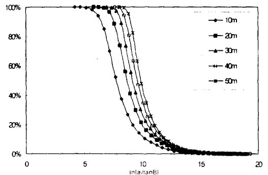
그림 4. 격자 크기변화에 따른 지형지수의 변화
