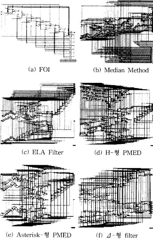
그림 13. Synopsys Design Analyzer를 이용한 합성 결과 Fig. 13. The results of the synthesis using the Synopsys Design Analyzer.
