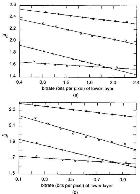
그림 5. 독립적 부호화율 배분방법 성능. 부호화율 12Mb/s, (a) PSNR, (b) 두계층에 발생된 비트량
