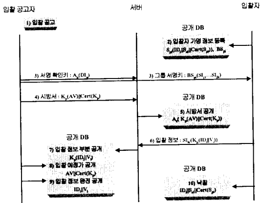
그림 3. 제안 방식 흐름도
