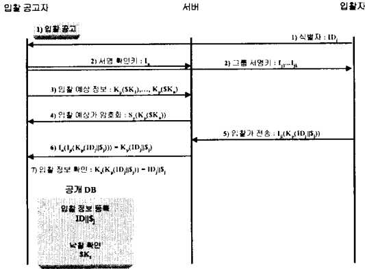
그림 2. PL 방식 흐름도
