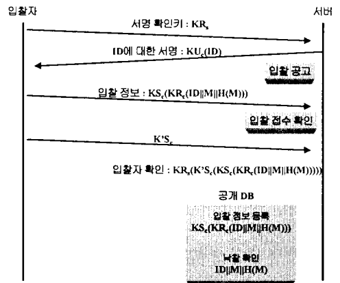
그림 1. LKR 방식 흐름도
