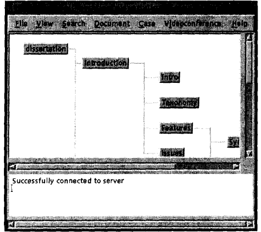
그림 4. 논리뷰
