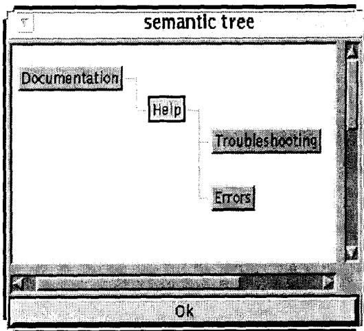
그림 7. 세만틱 네트워크
