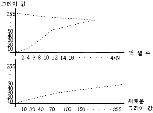
그림 5. 후보영역의 히스토그램과 LGT의 변환 특성
