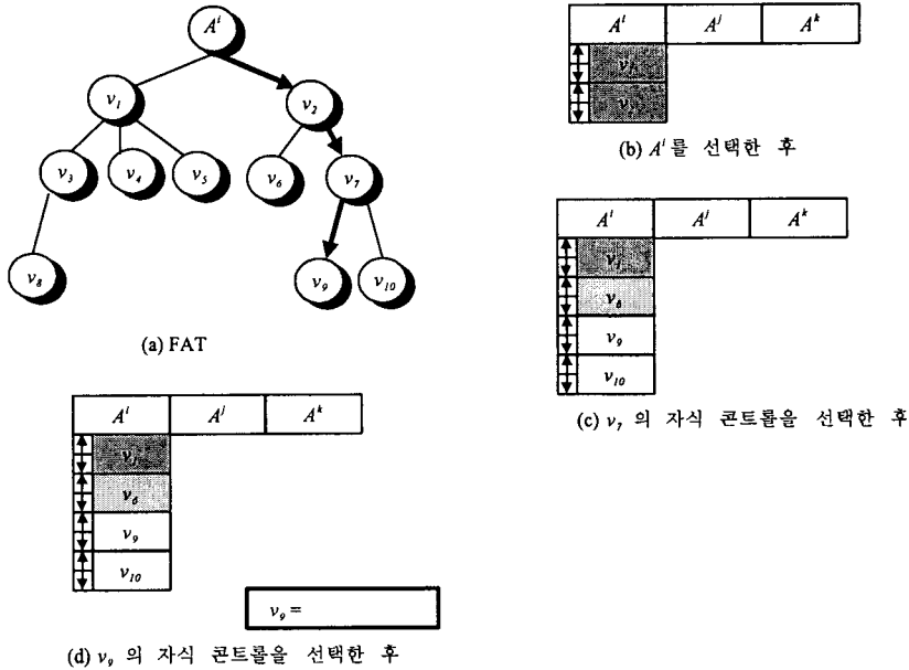
그림 2. FAT의 브라우징
