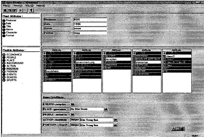
그림 3. 사진 브라우저
