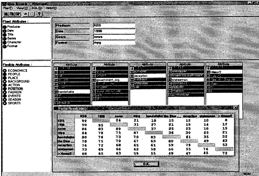
그림 5. 결과 브라우저
