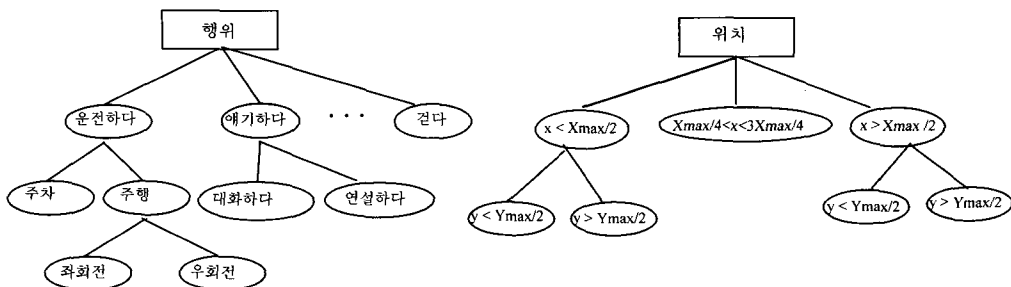
그림 1. FAT의 예
