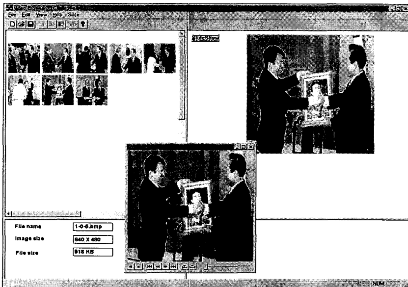
그림 4. 결과 뷰어
