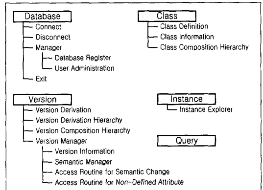
(그림 10) 전체 메뉴 구성
