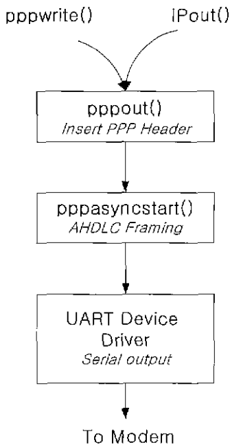
(그림 7) 임베디드 시스템의 PPP 출력 흐름도
