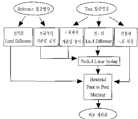
(그림 3) 시스템 구성도
