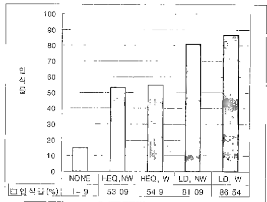
(NONE : 전처리 없음, HEQ : 히스토그램 평활화, LD : local difference, NW 가중치 없음, W 가중치 있음) (참조 이미지 개수 25개, 입력 이미지 개수 275개)
