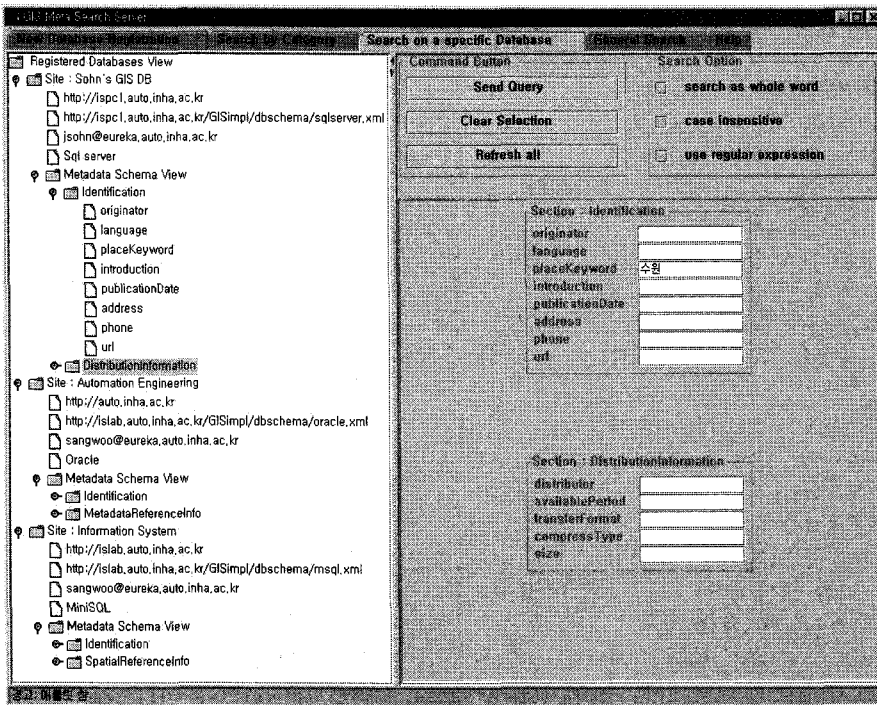
그림 14. 특정 GIS 데이터베이스에 대한 검색 인터페이스
