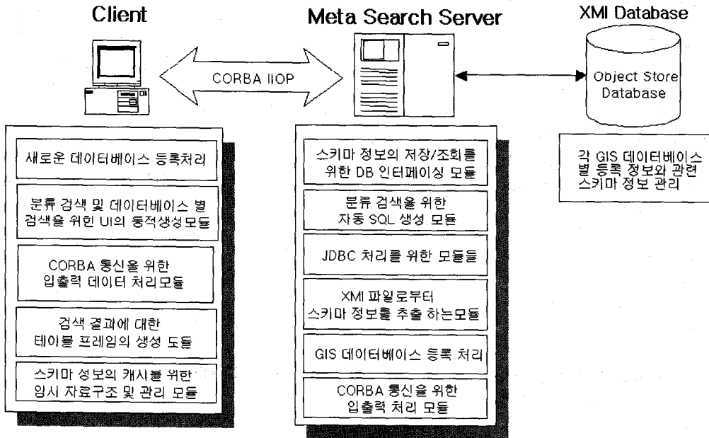
그림 5. 시스템의 주요 기능 및 모듈 구성
