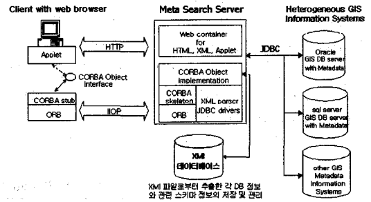
그림 4. 시스템 구성도
