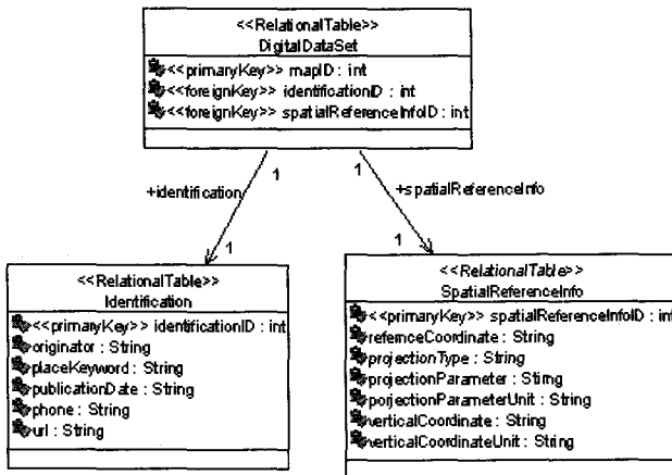
그림 10. MiniSQL GIS 메타데이터 스키마
