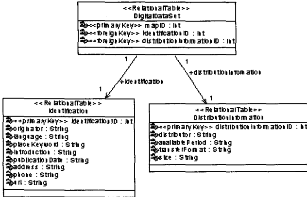
그림 8. SQL Server GIS 메타데이터 스키마
