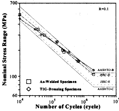
그림 3.1 공칭응력범위-반복횟수 선도
