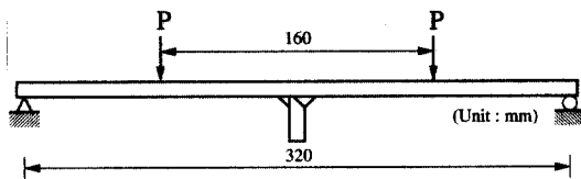
그림 2.3 피로실험방법
