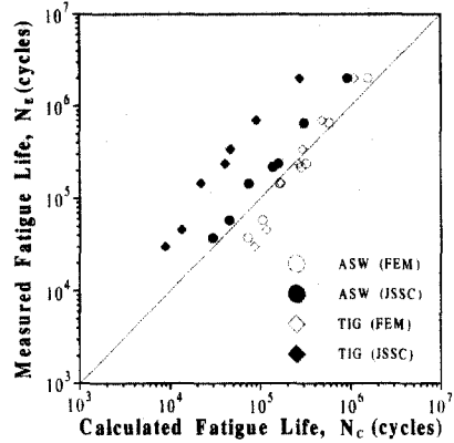
그림 5.6 실험피로수명과 계산피로수명과의 비교
