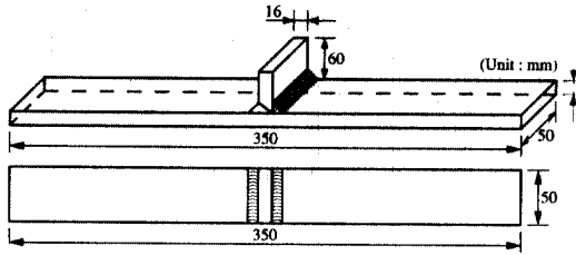
그림 2.1 시험체 형상 및 치수
