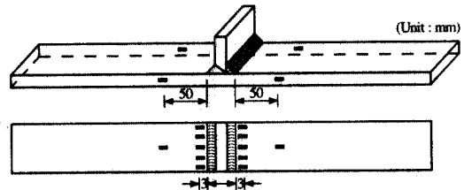
그림 2.4 변형률게이지 부착위치
