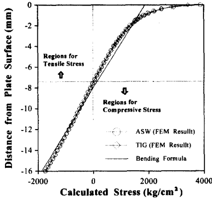
그림 4.4 판두께 방향의 응력분포도
