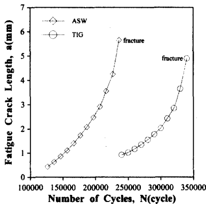
그림 5.3 균열길이(a)-반복회수(N) 선도
