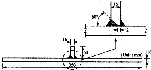
그림 2.2 시험체 용접모식도
