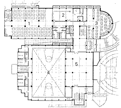
1층 평면도
