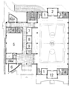
1층 평면도
