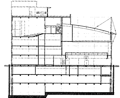
횡단면도
