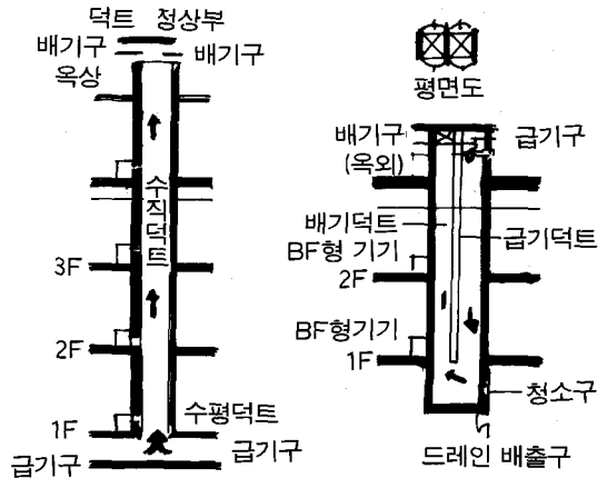
〈그림 3〉 SE 및 U덕트의 설치 예
