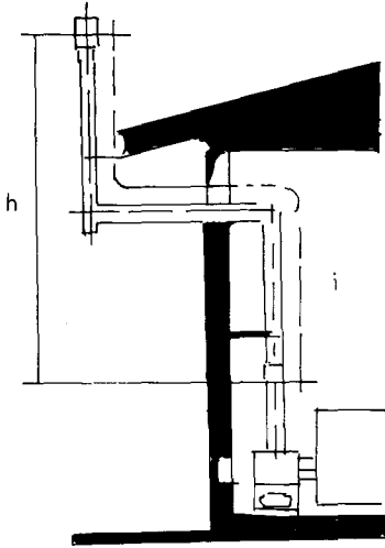
<그림 1> 배기통의 높이
