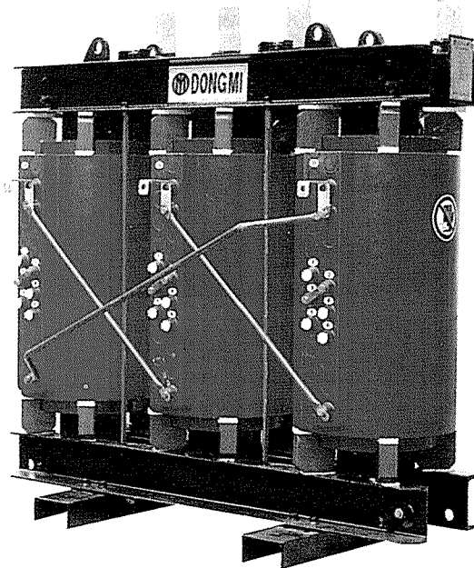
(진공 주형방식의 MOLD 변압기)
