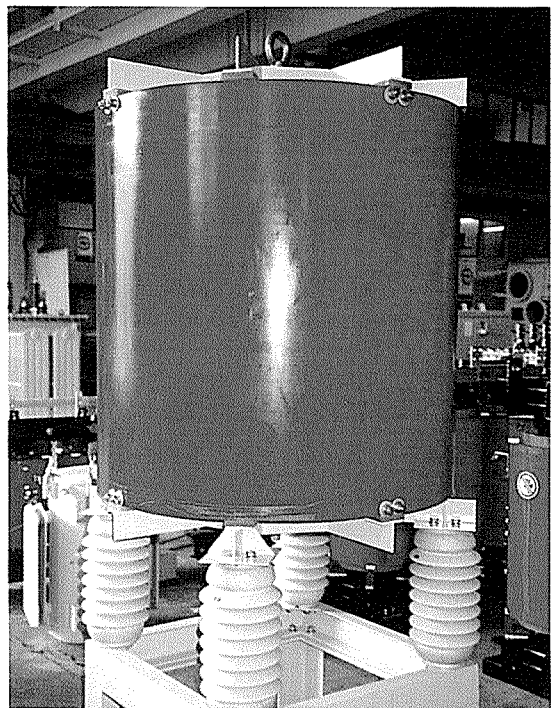
(22.9kV급 변압기 중성점 접지 리액터 모습)
