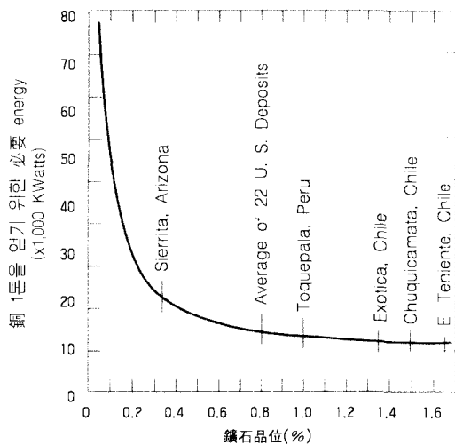
〈그림 8〉 동(Cu) 1톤 생산에 필요한 에너지와 광석품위와의 관계도(Page and Creasey, 1975)
