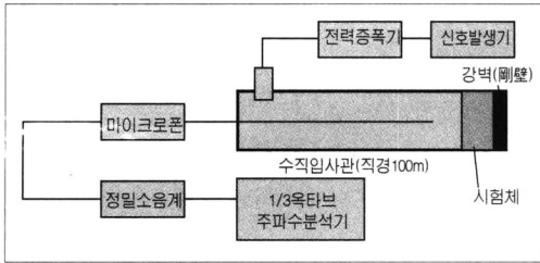
그림1 수직입사 흡음율시험장치 개요도
