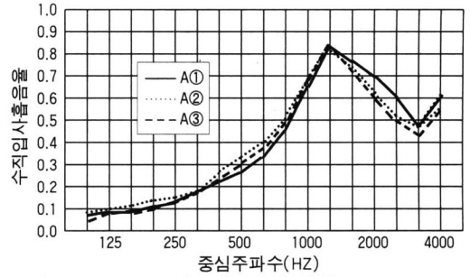
그림3 표면코팅처리의 영향
