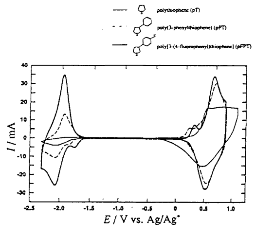
그림 6. 1M Et 4 NBF 4 /acetonitrile 용액에서 pT(가선), pPT(점선), pFPT(굵은 선)의 CV곡선.
