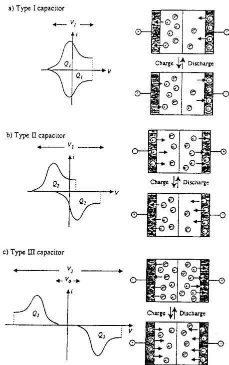
그림 4. 전도성 고분자를 전극으로 이용한 캐피시터의 충전 방전 메커니즘과 CV곡선.
