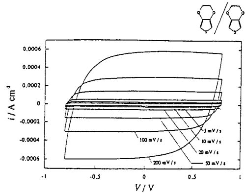
그림 5. LiClO 4 /acetonitrile 용액에서 다른 주사속도로 얻은 Poly(3,4-ethylenedioxythiophene)의 CV곡선.
