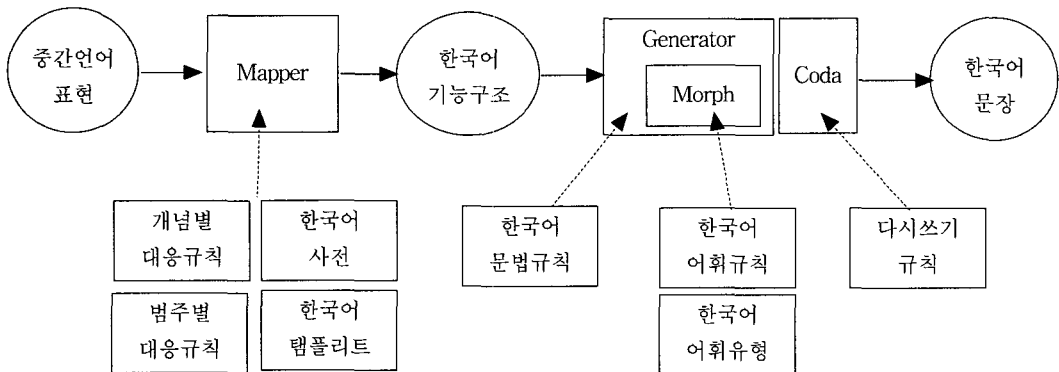
(그림 2) KANT 생성 시스템의 처리 절차
