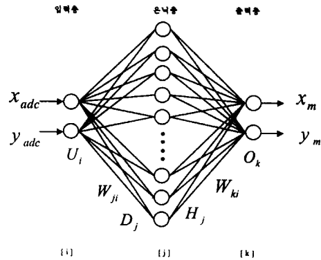
그림 3.2 신경 회로망의 구조 Fig. 3.2 Construction of neural network
