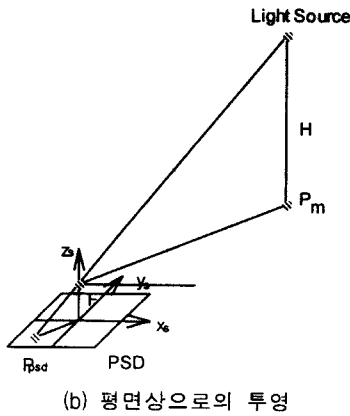
그림 3.1 PSD 센서 시스템 Fig. 3.1 PSD sensor system
