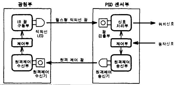
그림 2.2 PSD 센서 시스템 구성
