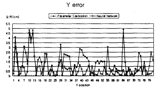
그림 4.4 파라미터 캘리브레이션과 신경 회로망에 의한 위치측정 오차 비교
