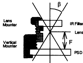
그림 2.1 광 검출부 Fig. 2.1 Light detector part
