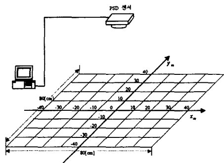
그림 4.2 PSD 센서 위치와 광원의 위치 Fig. 4.2 Position of PSD sensor and light source
