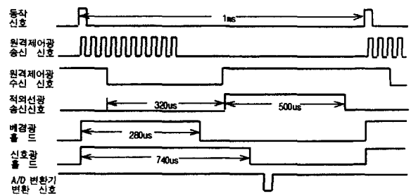
그림 2.3 PSD 센서 시스템의 동작 타이밍도
