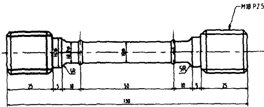
(a) Creep test specimen(ASTM E139-83)
