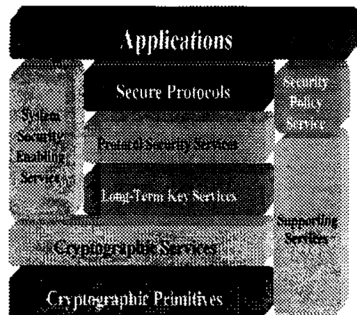
<그림 1> 공개키 기반 하부 구조
