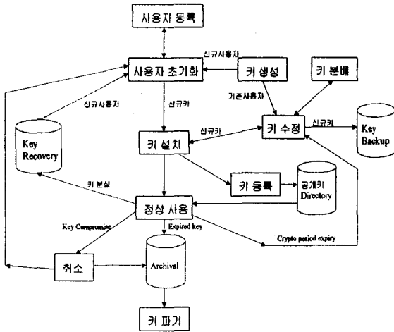
<그림 2> 키 관리 생명 주기
