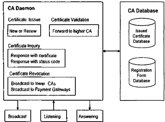
<그림 9> SET에서의 인증 구조
