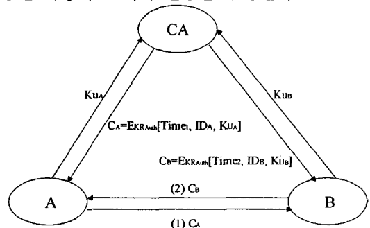
<그림 3> 공개키 기반 인증기관 인증 정보흐름
