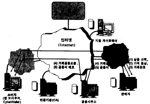
<그림 6> 구매작업, 거래 완료 및 거래내역 공증
