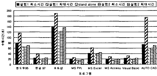
그림 5. 네트워크 장비에 따른 DL-NCS의 성능 비교
